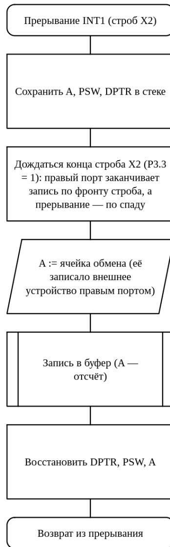
Рис. 3.6. Схема алгоритма: Обработчик прерывания INT1: приём отсчёта X2 от внешнего устройства
